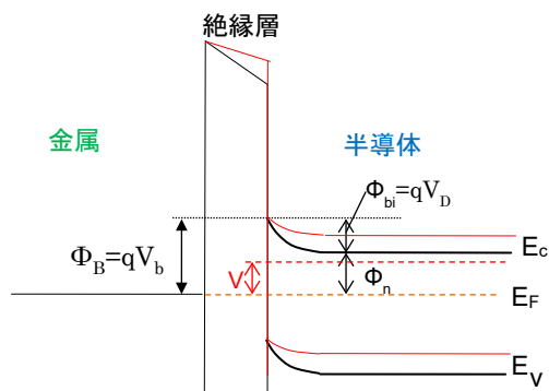
図 12 MIS ショットキーダイオードの順バイアス時のバンド変化 黒線が無バイアス時 赤線がバイアス印加時を表す。界面層と界面準位を仮定した n 型 Si と金属のショットキー接合のバンドモデルである
