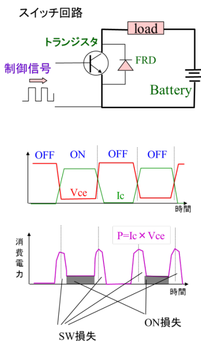
図 11 スイッチ回路における ON 損失と SW 損失
