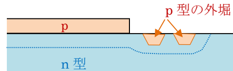
図9 ガードリング構造
