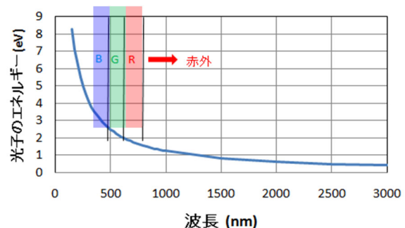
図 20 光のエネルギーと波長の関係 半導体においては、バンドギャップ以上
