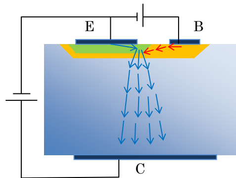
図 11 実際のトランジスタの断面図と ON 動作のときの電子(青線)とホール(赤線)の流れ この図は npn トランジスタの例
