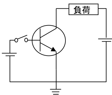
図 15 スイッチトランジスタとしてのバイポーラトランジスタの使用事例
